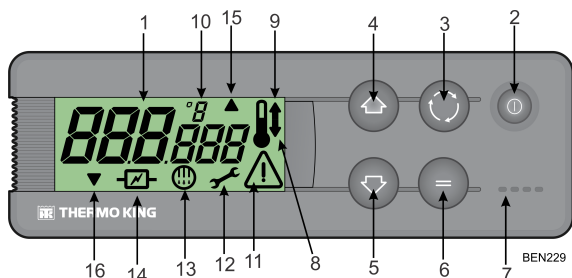
Рис. 9. Дисплей внутрикабинной панели управления (НМИ), кнопки, символы
