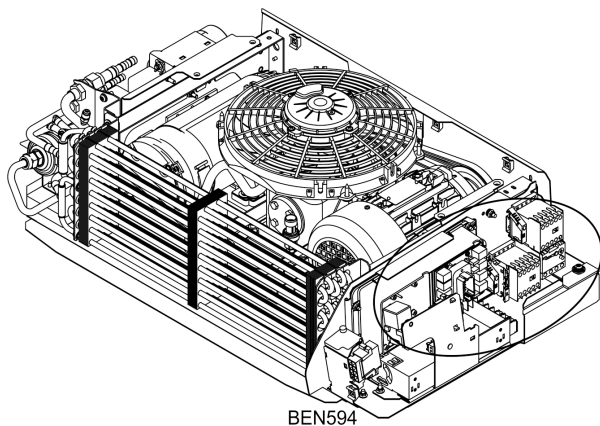
Рис. 11. Расположение предохранителя (крышка конденсатора снята)
